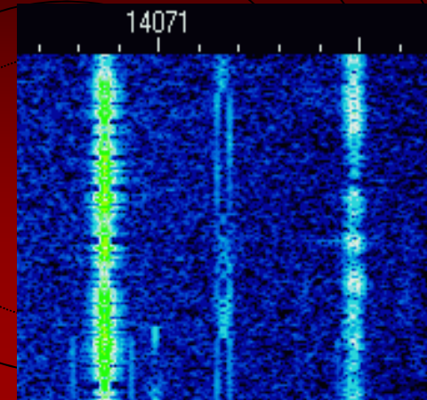
PSK31 Trace
